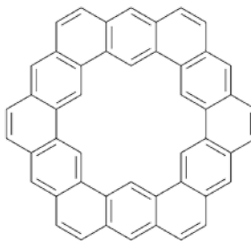
Кекулен
