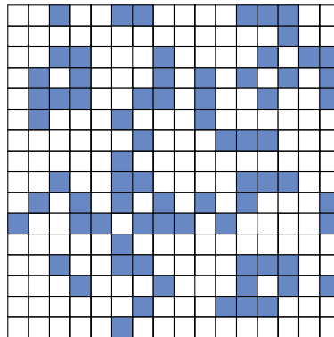
Суперключ, открывающий все двери 2^k \times 2^{5-k} , k = 1, 2, 3, 4
