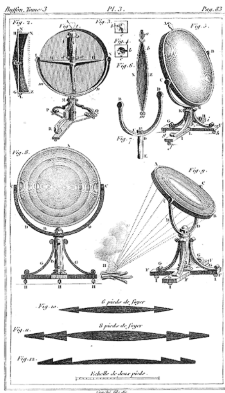
Рис. 2. Бюффон предлагал вытачивать линзу сложной формы целиком. Одна из линз собирает пришедшие от Солнца параллельные лучи и поджигает расположенный в фокусе хворост
