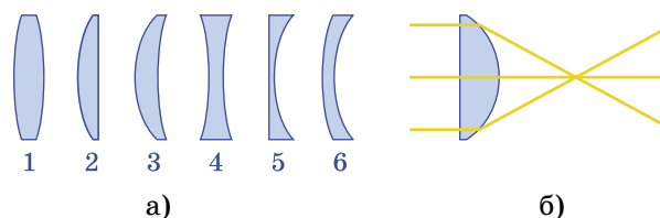
Рис. 1. а) Разные виды выпуклых и вогнутых линз; б) плоско-выпуклая линза собирает параллельные лучи в фокусе
