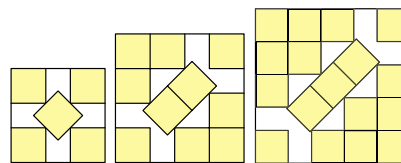
Рис. 2. Упаковки Гёбеля для N=5, 10, 17 (первые две оптимальны, последняя нет)
