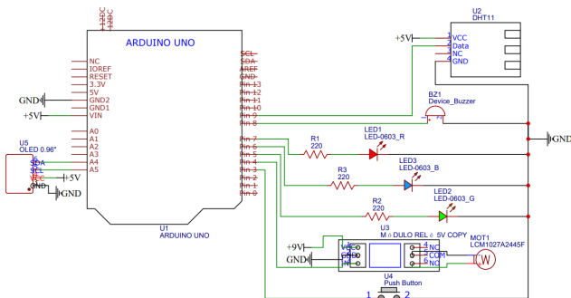
Figure 5. Esquema de Conexión Reto 3
