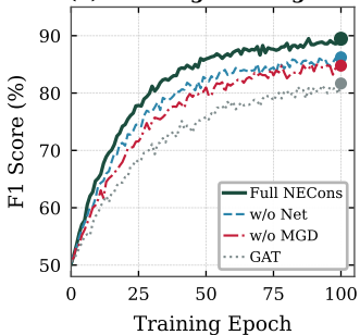
(d) Training Convergence
