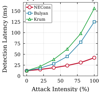
(d) Detection Latency
