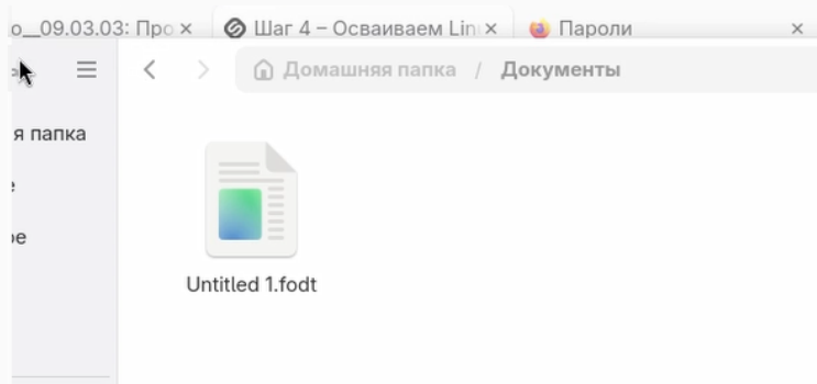
Рис. 6: Создание файла
