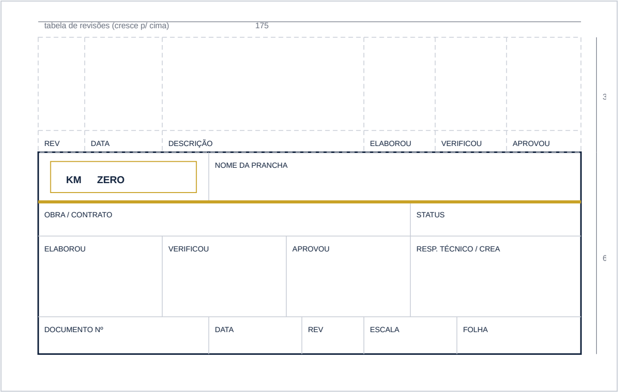
Figura 1 — Carimbo 175 × 65 mm com a zona reservada à tabela de revisões. Cotas em mm, escala livre. Fonte: KMZERO, 16/09/2026.
