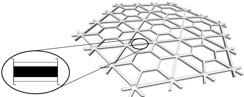
Tensar NX850 Geogrid Vista en perspectiva
