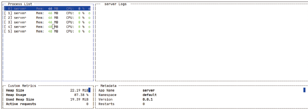
▼ 그림 15-5 npx pm2 monit 명령 실행 화면
