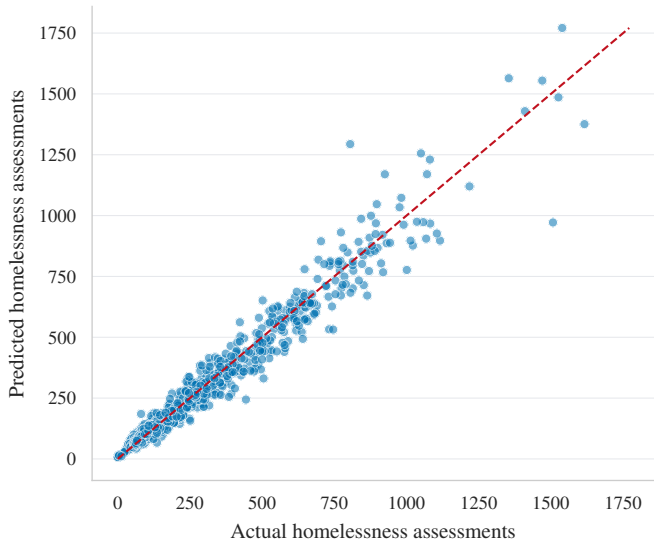
Actual vs predicted, test (correlation = 0.978)
