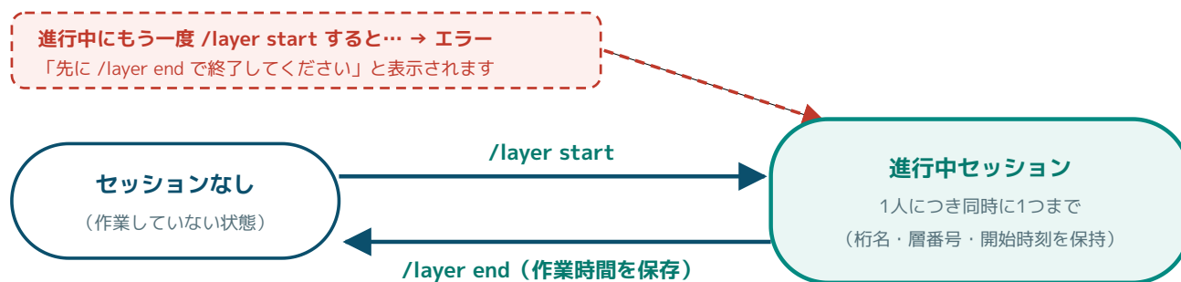
図2 セッションの状態遷移：start 中にもう一度 start はできない
