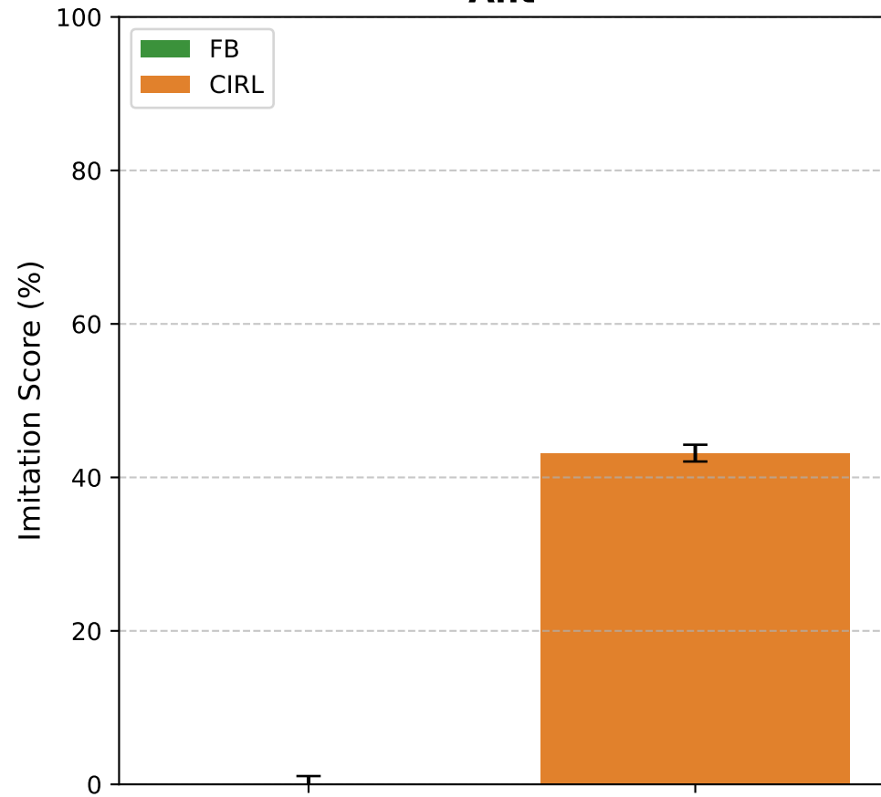
Ant
