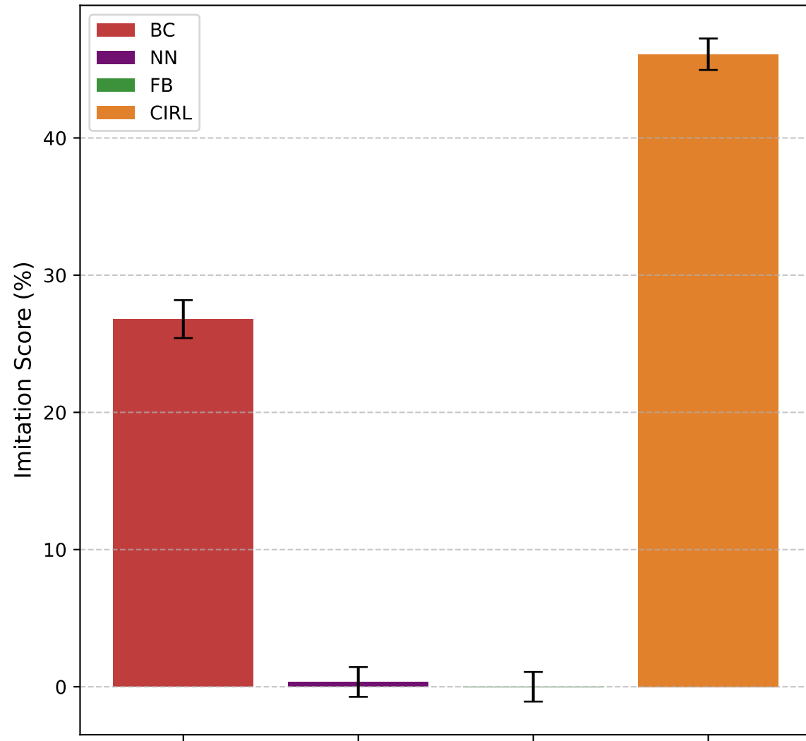
Ant
