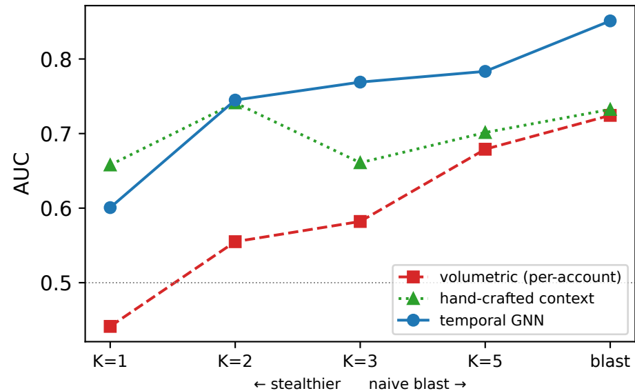
AUC
