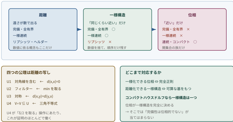
図30-1 距離・一樣構造・位相の三層。一樣構造は距離から数値を捨てて順序関係だけを残したもので、完備性と一樣連続性はこの層に属する。
