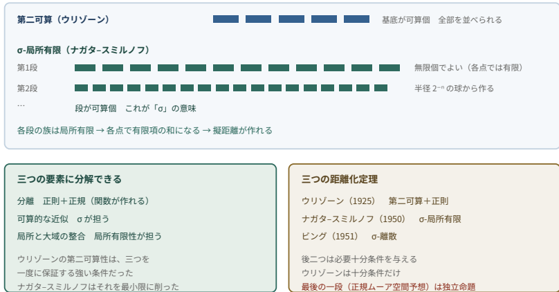
図32-1 可算基底を「可算個の局所有限な族」に置き換える。各段が局所有限なので、無限個の関数の和が各点で有限項に落ち、擬距離が作れる。
