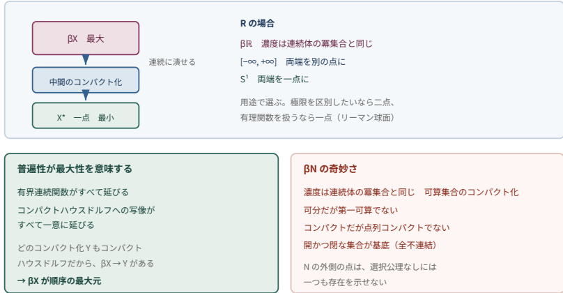
図23-1 コンパクト化には順序があり、一点コンパクト化が最小、ストーン-チェックが最大である。 \beta\mathbb{N} は可算集合のコンパクト化でありながら、濃度も構造も極端に大きい。
