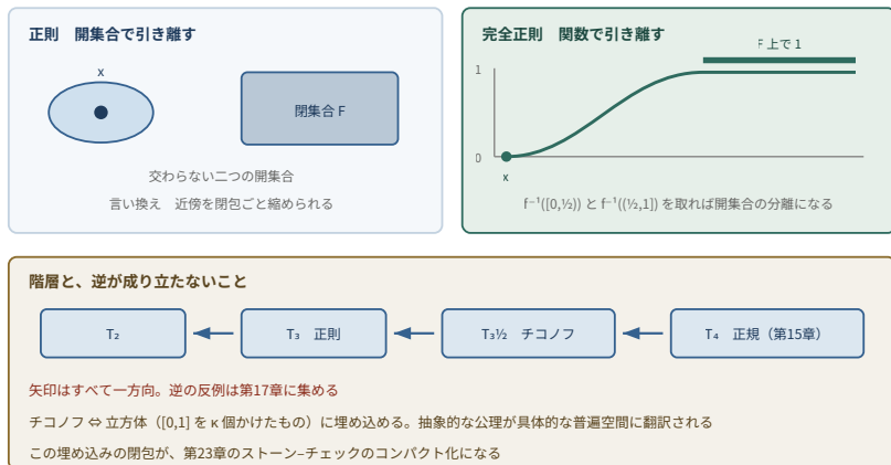
図14-1 正則性は開集合による分離、完全正則性は連続関数による分離。後者のほうが強く、立方体への埋め込みという具体的な特徴づけをもつ。
