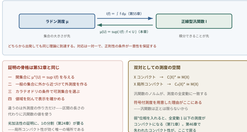
図59-1 測度から積分を作る道と、積分から測度を作る道は、同じ理論の二つの入り口である。リースの表現定理は両者を一対一に対応させ、測度の空間を連続関数の空間の双対として位置づける。
