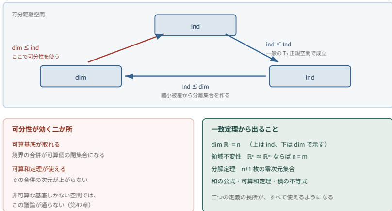
図41-1 三つの不等式を環状に示す。dim ≤ ind の一歩でだけ可分性が要る。一致すると、三つの定義それぞれの長所が同時に使えるようになる。
