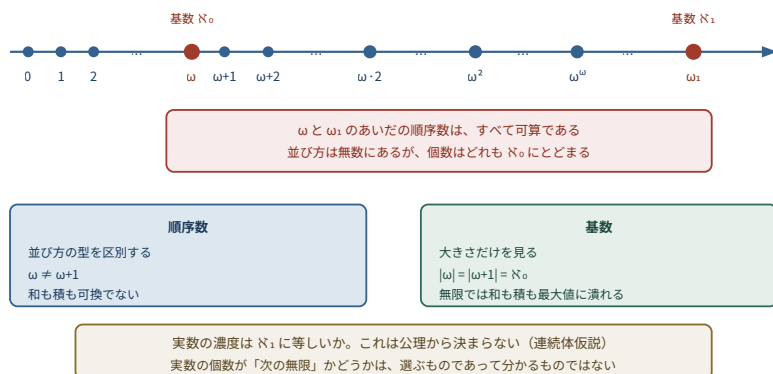
図4-1 順序数は並び方を、基数は大きさを表す。可算な順序数は \omega_1 の手前に無数に並び、どれも濃度は \aleph_0 である。
