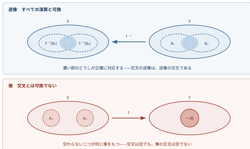
図2-1 逆像は一点ごとの条件に還元されるので、合併・交叉・補集合のすべてと可換になる。像は存在の主張なので、交叉が潰れる。連続性を逆像で定義するのは、この非対称のためである。
