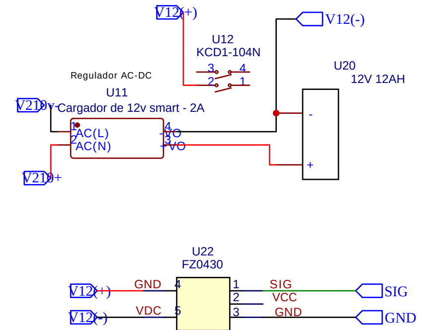
MODULO 1- ENERGIZAR CIRCUITO
