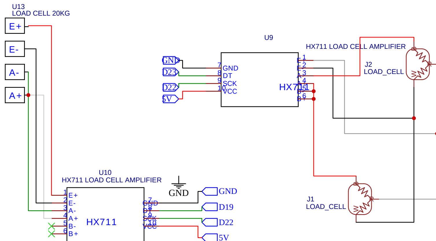
MODULO 2- SENSOR PRESIÓN
