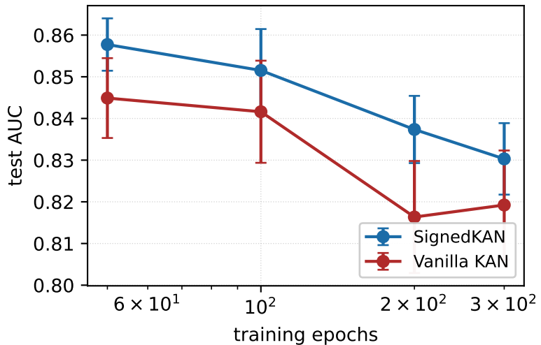
Bitcoin OTC
