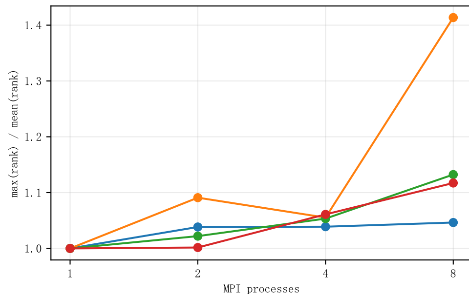
Kunpeng PBS: load balance
