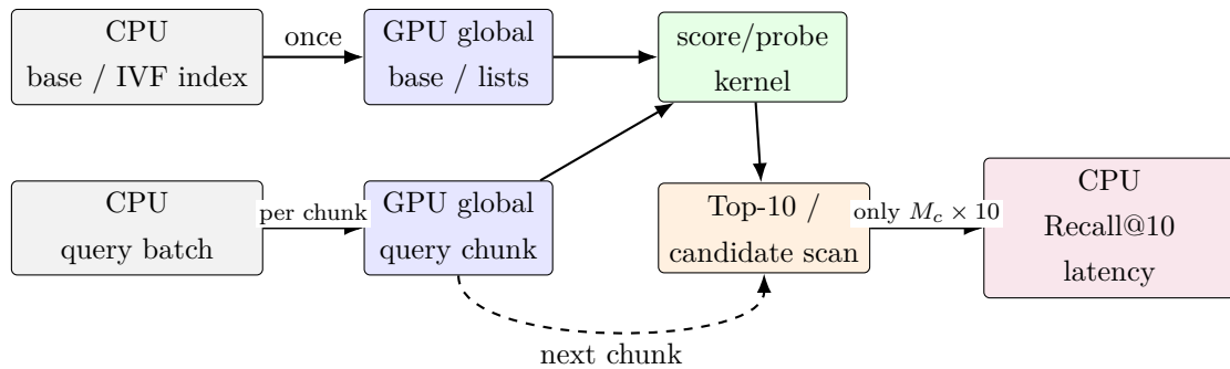
图 2 CUDA batch ANN 搜索的数据流与阶段划分
