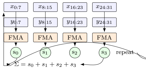
图 3.2 Flat-AVX2 四累加器点积的数据流：每组 8-float 向量块的 FMA 与累加器彼此独立，循环内无跨块依赖，归约推迟到循环结束后
