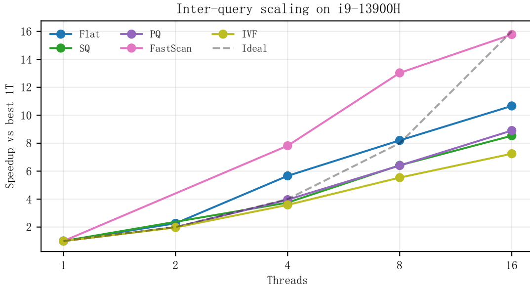
图 6 本地 i9 上 inter-query 的多线程加速比，基准为同算法最优 1 线程配置
