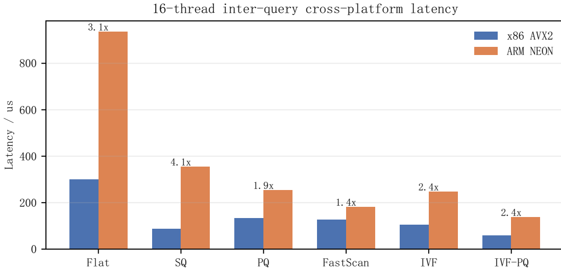
图 12 16 线程 inter-query 下 x86 AVX2 与 ARM NEON 的延迟对比
