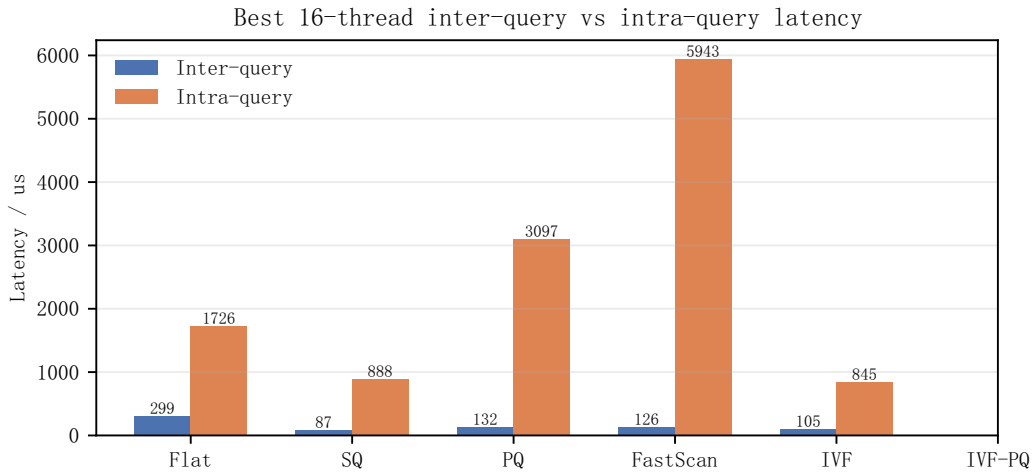
图 7 本地 16 线程下 inter-query 与 intra-query 的最优延迟对比 (IVF-PQ 的 intra 数据因 local 模式下 intra 实现未覆盖而缺失，鲲鹏侧 IVF-PQ local intra t=16 为 1630 \mu s ，比 inter 的 141 \mu s 慢 11.5 \times )
