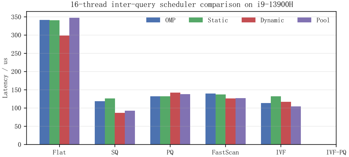
图 8 本地 16 线程 inter-query 下 Pthread / OpenMP 调度策略对比
