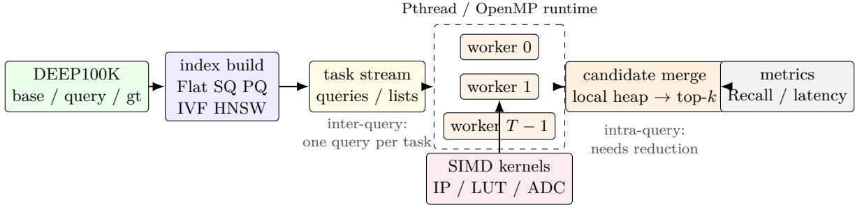
图 1 ANN 多线程检索流水线：索引结构决定单次搜索的工作量，线程层决定任务如何分配，SIMD 内核决定每个 worker 的距离计算常数
