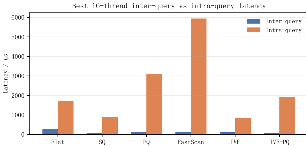
图 6 本地 16 线程下 inter-query 与 intra-query 的最优延迟对比
