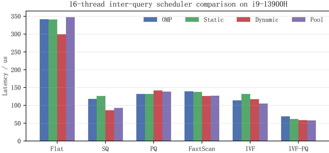
图 7 本地 16 线程 inter-query 下 Pthread / OpenMP 调度策略对比
