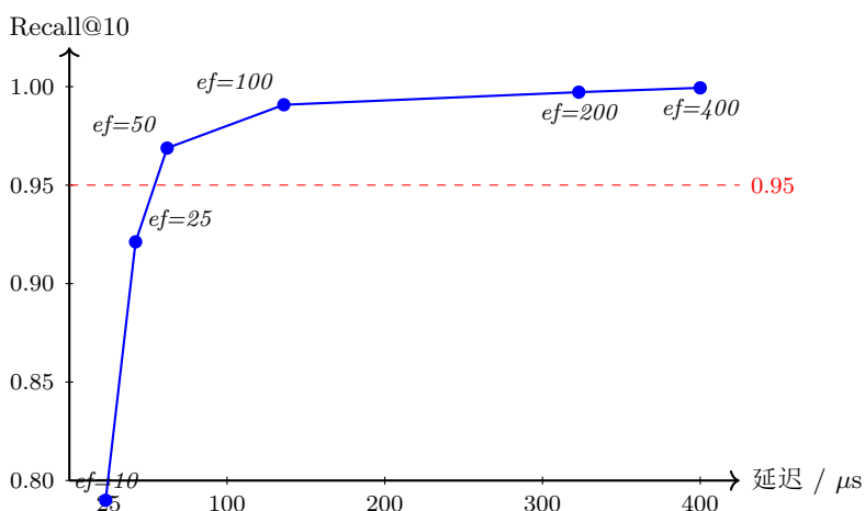
图 10 HNSW ef sweep 的 recall-latency 曲线。ef=50 是过 0.95 准入门槛后延迟最低的设置，ef=100 给出 0.99 高召回但延迟约 2.2 \times ，ef=200 之后 recall 收益快速饱和
