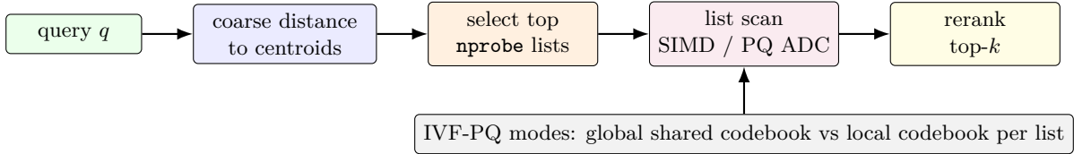
图 4 IVF / IVF-PQ 的 coarse-to-fine 检索流水线
