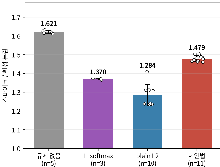
(F5) 살아남은 뉴런이 얼마나 세게 쏘나 제안법 - plain L2: t=10.5 , p=8.4e-07
