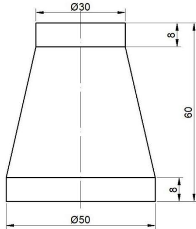
图5初赛的物料形状
