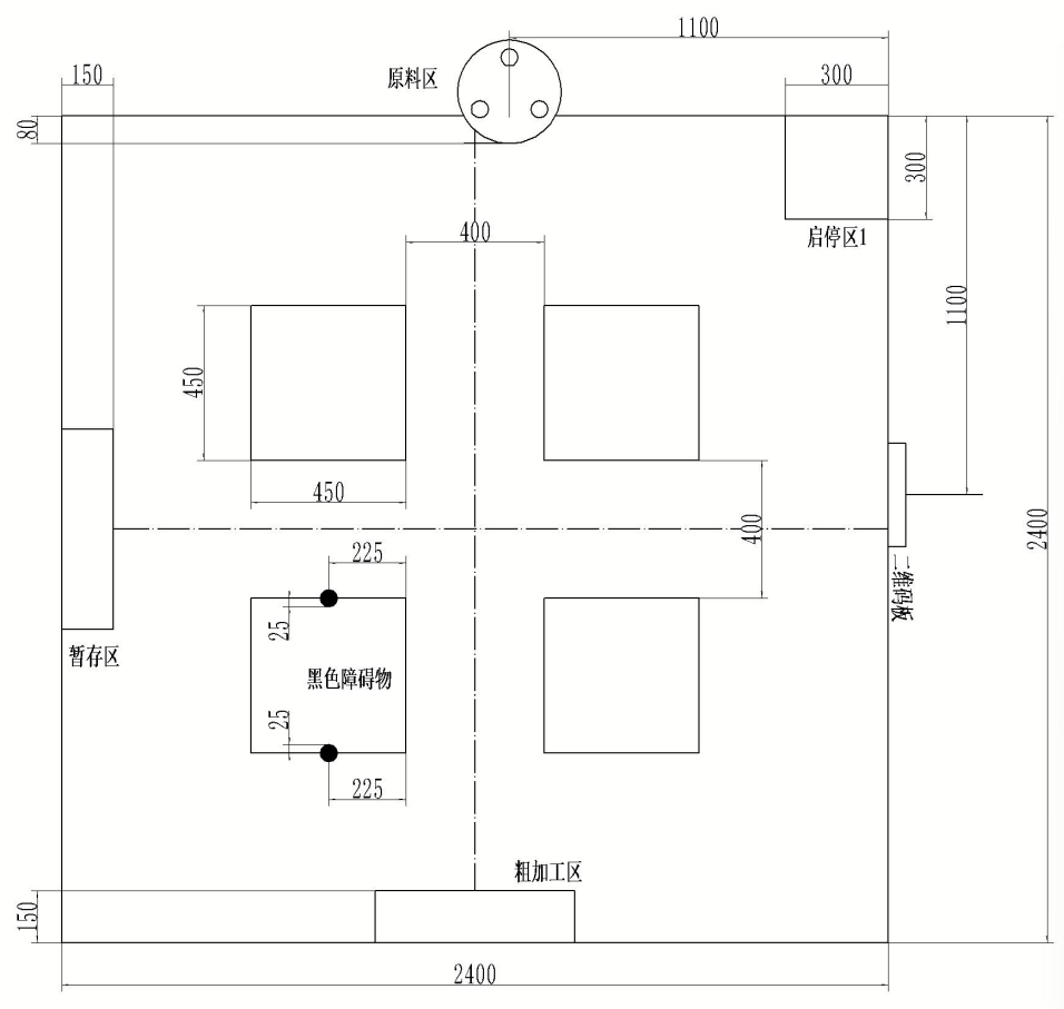
图6现场初赛场地示意图
