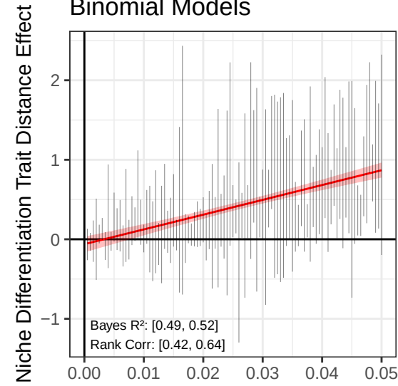
Binomial Models
