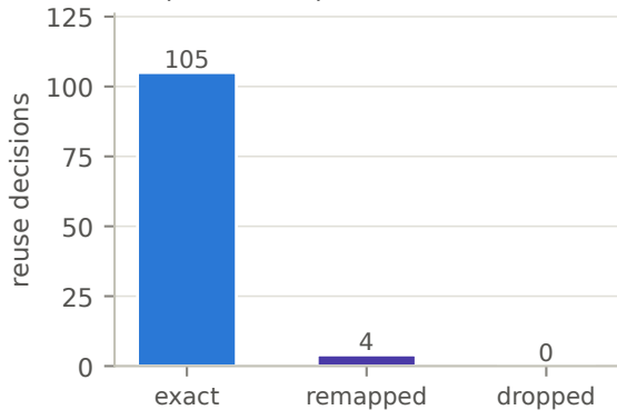
Temp-0 run (60 plans)
