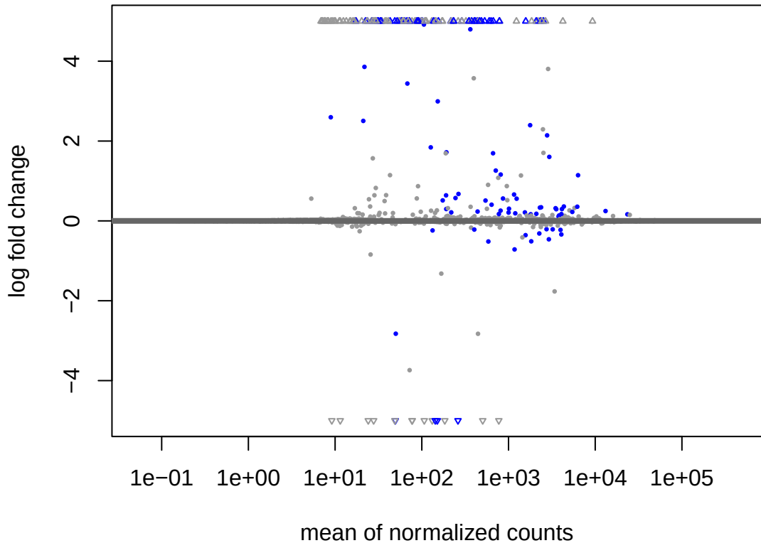
MA Plot: HT_F vs WT_F
