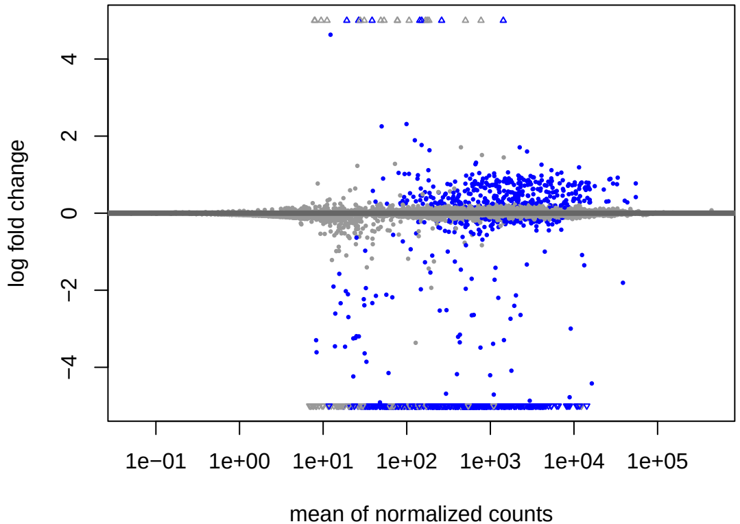
MA Plot: KO_M vs HT_F
