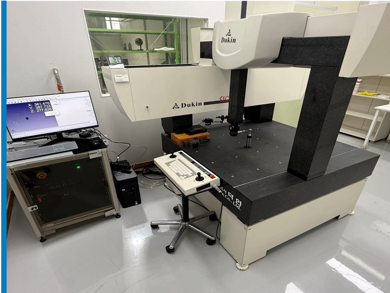
3차원 측정실
