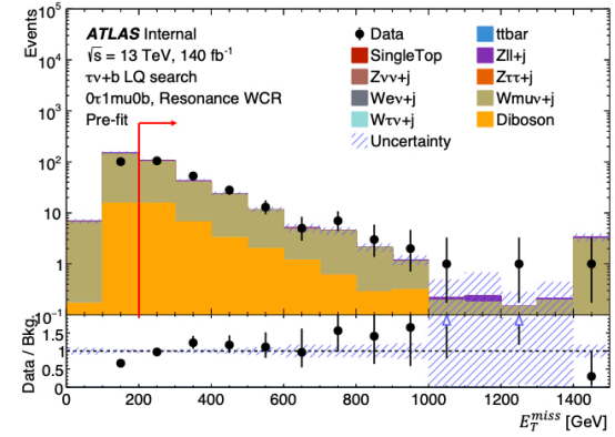
(d) E_T^{miss} , \mu channel
