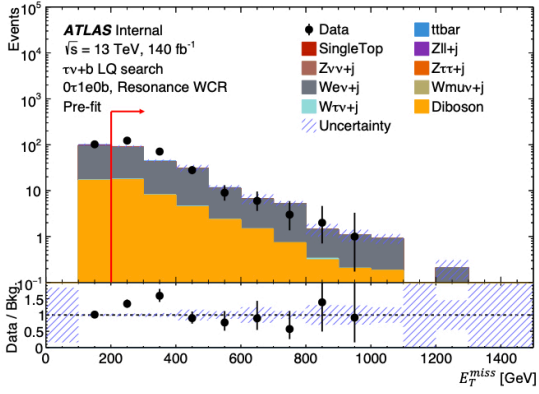
(c) E_T^{miss} , e channel
