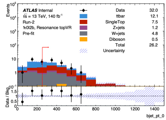
(d) p_T^b
