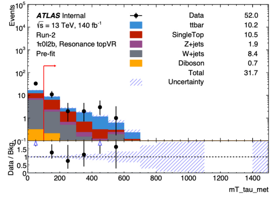
(b) m_T
