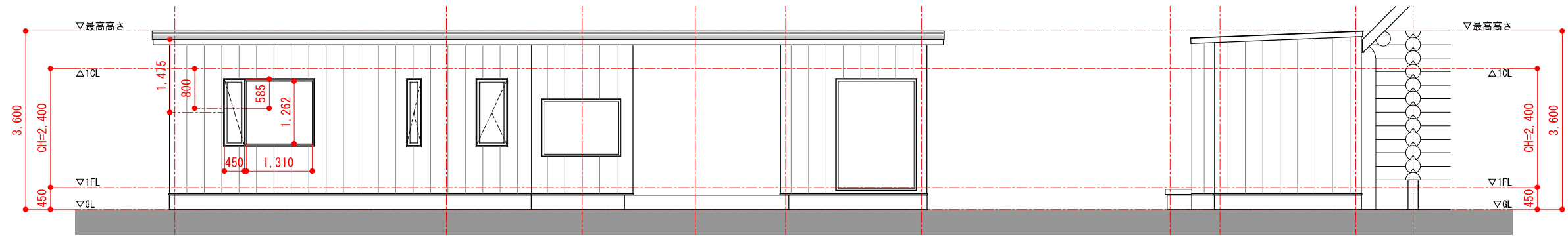
北側立面図 1 : 100
