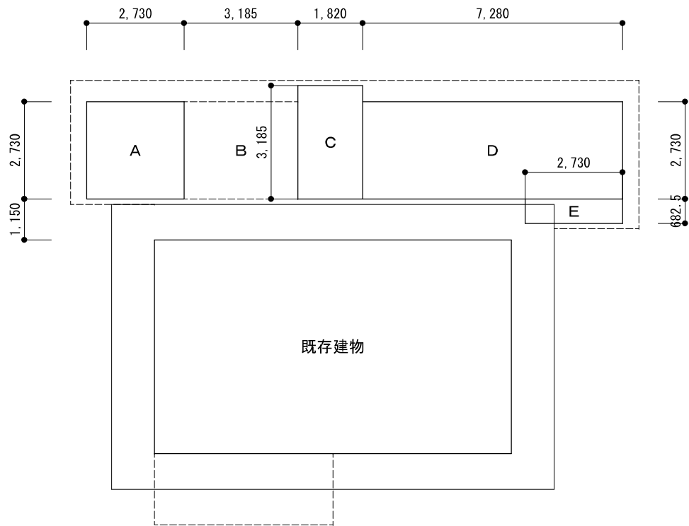
1 階求積図 1 : 150
