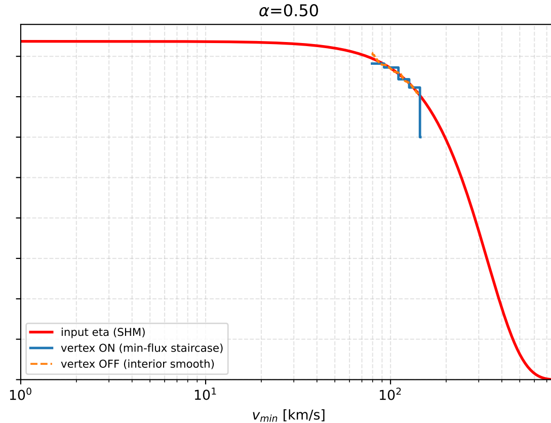
Vertex ON vs OFF - M1 (10 MeV), TES Al q0 R5 SHM
