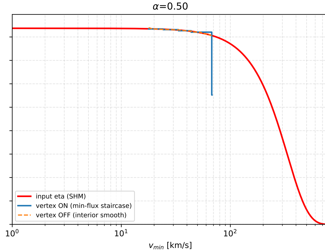
Vertex ON vs OFF - M2 (100 MeV), TES Al q0 R5 SHM
