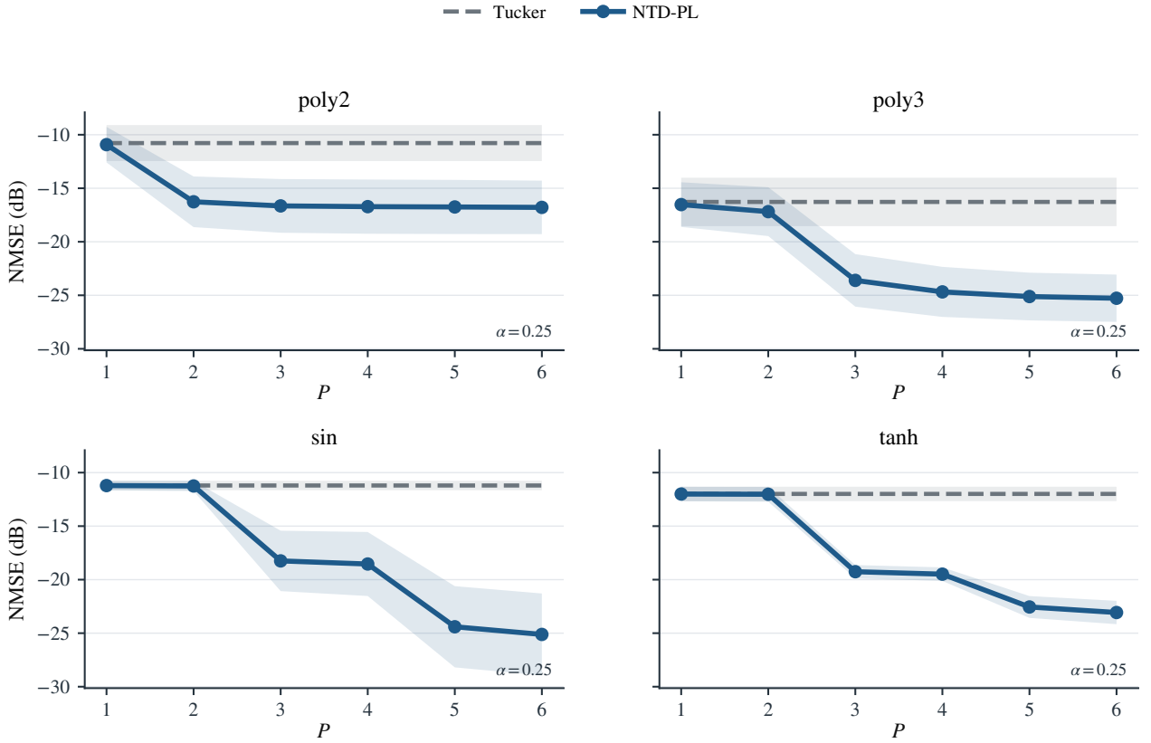
图 2: 固定非线性强度下, NTD-PL 的逼近误差随多项式最高阶数 P 的变化, 并与 Tucker 对照。图中显示 P=1 与 Tucker 接近 (线性一致性), 随后随 P 增大误差下降且边际收益逐步趋于饱和。
