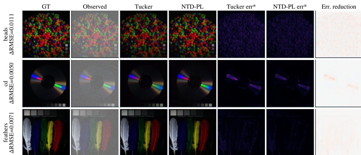
图 13: CAVE 随机缺失补全的代表性空间可视化。各列依次为原图、带掩膜的观测输入、Tucker 补全、NTD-PL 补全、Tucker 的 missing-only 误差、NTD-PL 的 missing-only 误差，以及 missing-only 误差下降图。最后一列按 Tucker – NTD-PL 定义，正值表示 NTD-PL 在缺失位置上进一步降低了补全误差。该图用于补充正文第 5.3.3 节关于“收益主要发生在缺失区域本身”的讨论。
