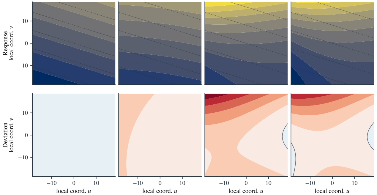
图 12: 固定二维 Tucker 局部 patch 时, 不同多项式最高阶数 P 下学习到的局部响应图与相对 P = 1 的偏差图。上排展示局部响应, 下排展示相对线性基线的偏差。该图用于补充正文第 5.2.2 节关于“新增表达能力如何随阶数逐步进入局部响应结构”的讨论。
