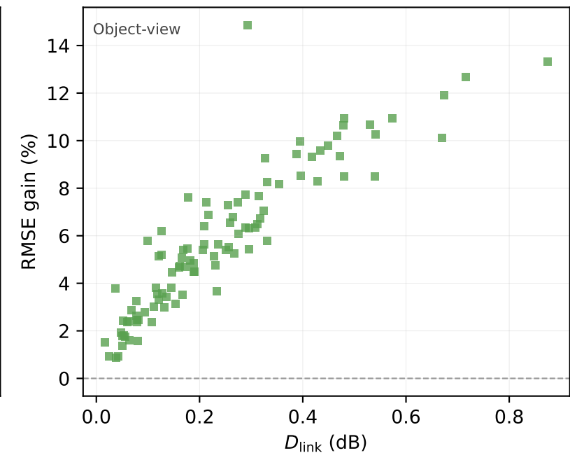
UCF101
