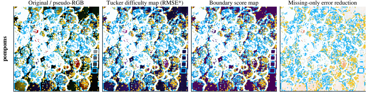
图 10: 代表性场景上的局部收益定位。四列依次为 pseudo-RGB 原图、Tucker 的 difficulty map (以缺失位置上的 RMSE* 定义)、boundary score map, 以及 NTD-PL 相对 Tucker 的 missing-only error reduction map。黄轮廓表示 top difficulty 区域, 青轮廓表示 top boundary 区域, 白轮廓表示两者的交叉区域。图中可以看到, 正增益主要集中在高难度与强边界同时出现的位置, 说明 NTD-PL 的补全优势具有明确的空间定位。
