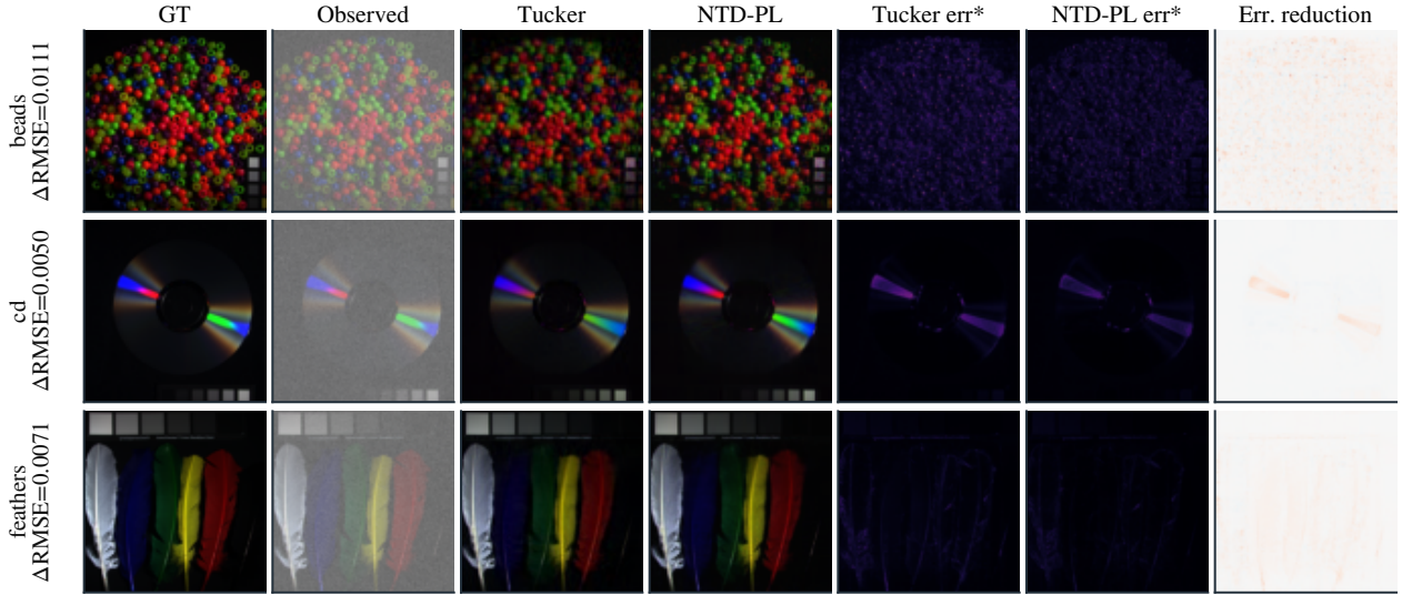
图 7: CAVE 随机缺失补全的代表性空间可视化。各列依次为原图、带掩膜的观测输入、Tucker 补全、NTD-PL 补全、Tucker 的 missing-only 误差、NTD-PL 的 missing-only 误差，以及 missing-only 误差下降图。最后一列按 Tucker – NTD-PL 定义，正值表示 NTD-PL 在缺失位置上进一步降低了补全误差。
