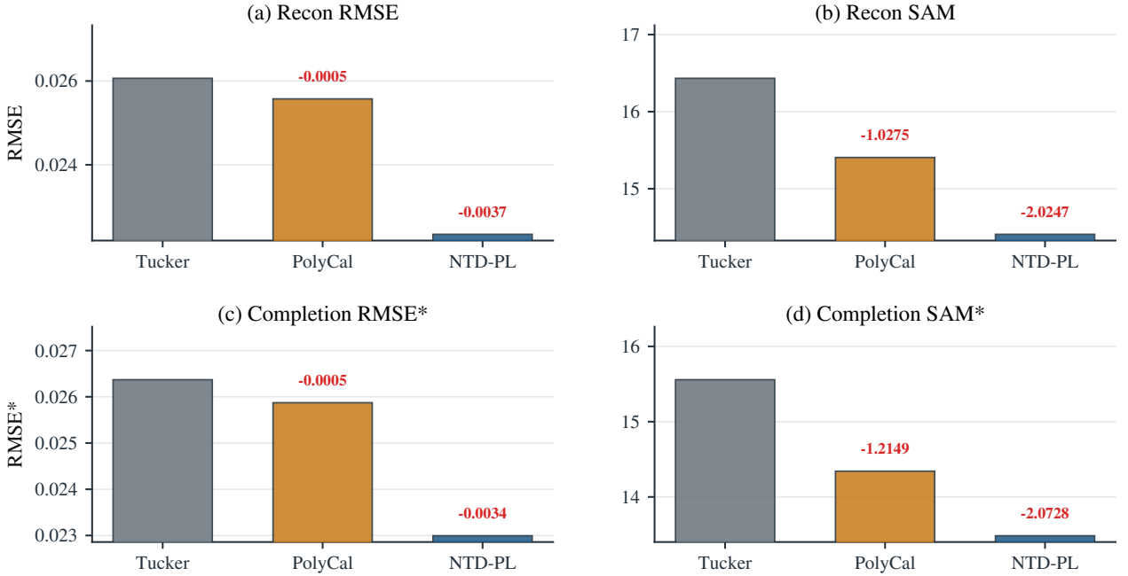
图 8: 机制区分主图。四个 panel 分别比较全观测重构的 RMSE、SAM 以及 \rho = 0.5 补全的 RMSE*、SAM*。三种方法都呈现出一致改进关系, 说明后处理只能部分逼近 NTD-PL 的收益, 而无法替代其联合建模。
