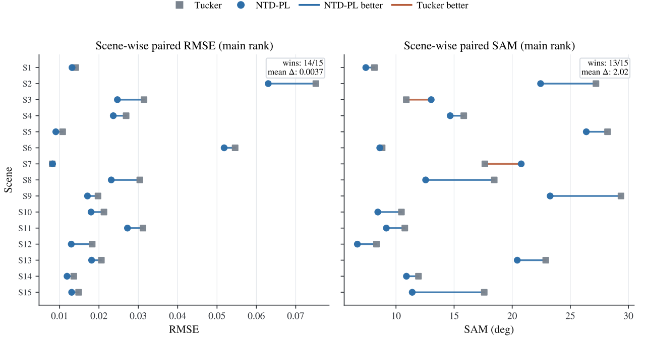
图 4: CAFE 全观测重构的场景级对比可视化。每条连线连接同一场景下 Tucker 与 NTD-PL 的结果；整体上，大多数场景都朝 NTD-PL 更优的一侧移动，说明其优势在场景层面具有一致性。
