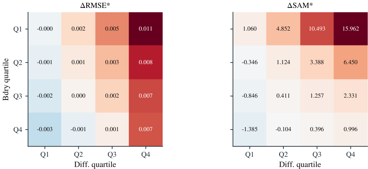
图 9: NTD-PL 相对 Tucker 的局部收益在困难 quartile 与边界 quartile 上的二维分布，正值表示 NTD-PL 更优。可以看到，收益并非均匀分布，而是主要集中在困难与边界的交叉区域。
