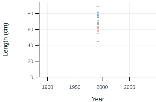
TR.EPO.2abc
