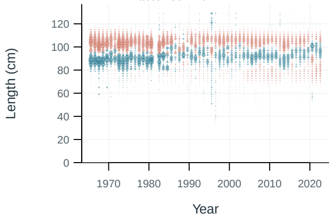
LL.INDEX.1abcd.1954-2022
