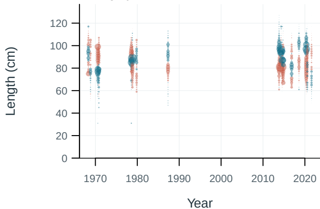
LL.EPO.2c
