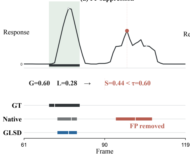
(a) FP suppression
