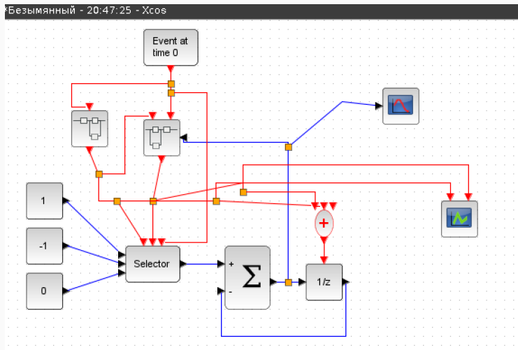
Рис. 5: Сама модель M|M|inf в xcos.
