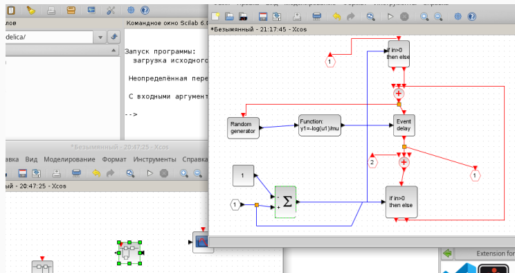
Рис. 4: Суперблок, моделирующий обработку заявок.
