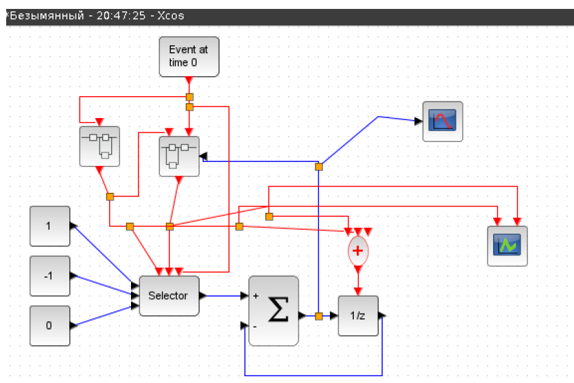
Рис. 6.1: Сама модель M|M|inf в xcos.
