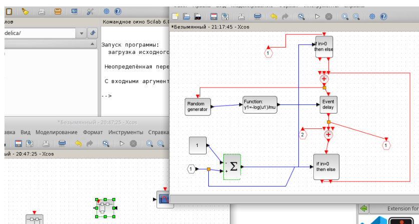
Рис. 5.1: Суперблок, моделирующий обработку заявок.
