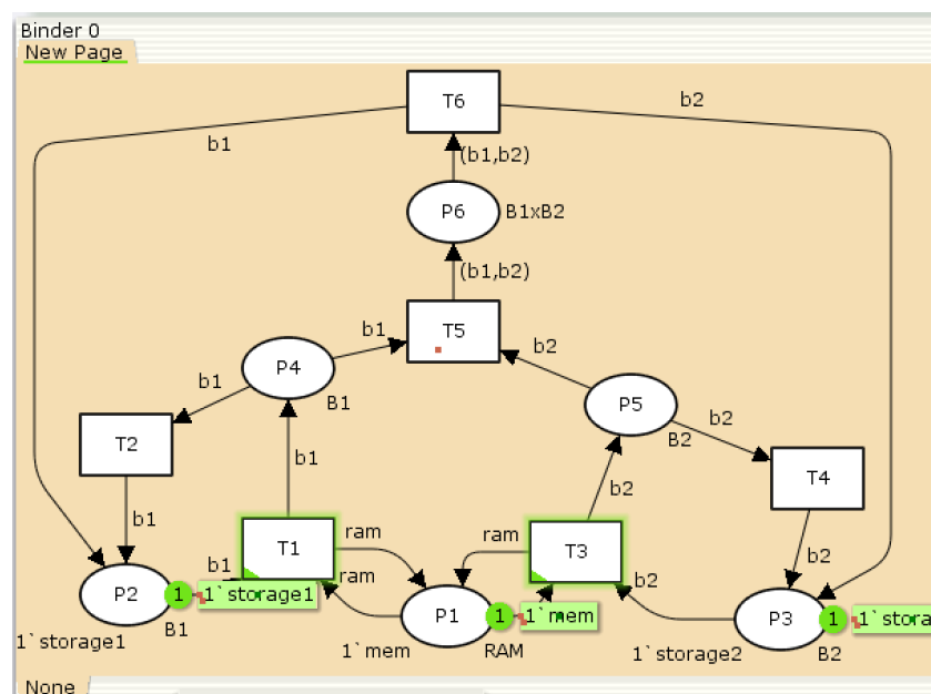
Рис. 2.1: Модель в CPN Tools.
