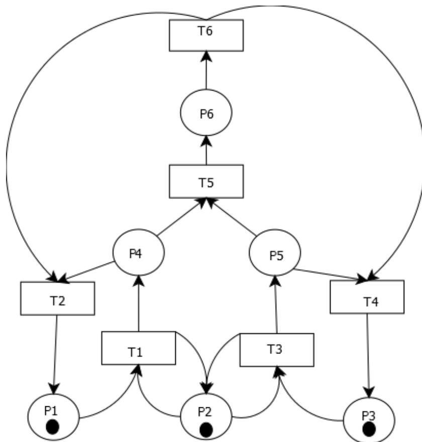
Рис. 4.1: Схема модели.
