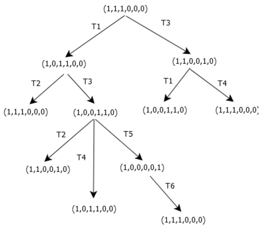
Рис. 5.1: Дерево достижимостей.
