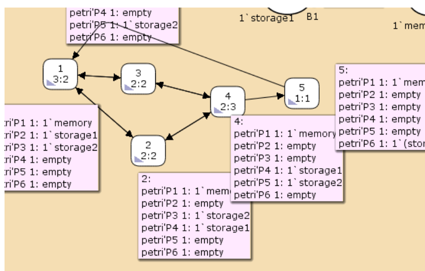
Рис. 6.1: Гра пространства состояний.
