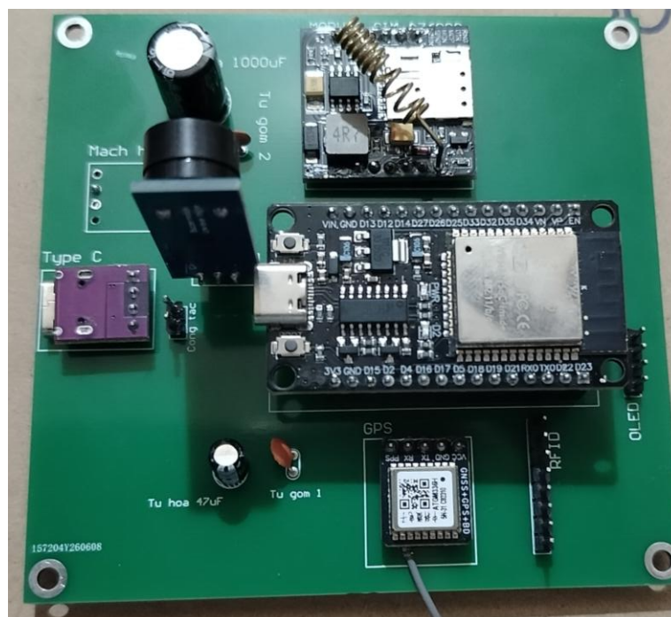
Hình 3.17 Mạch PCB sau khi hàn linh kiện
