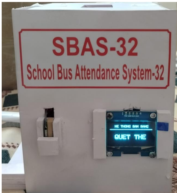
Hình 3.18 Mặt trước của hộp
