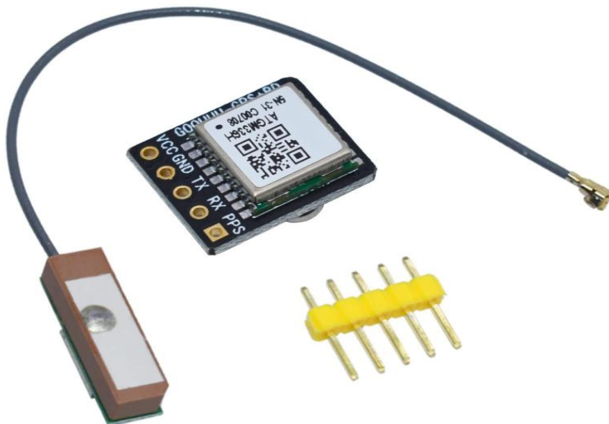
Hình 3.3 Module GPS ATGM336H
