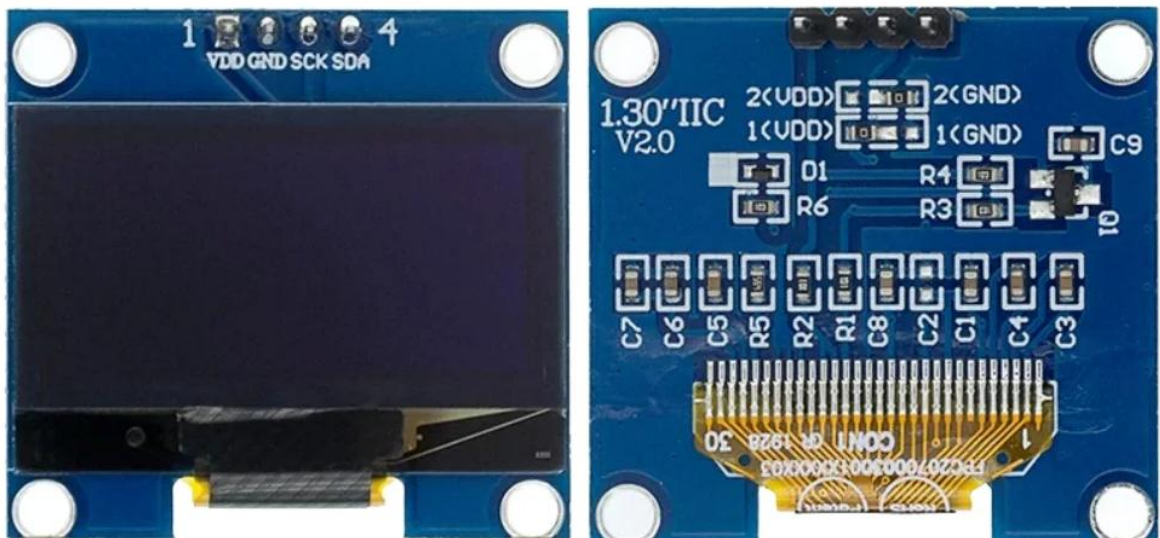
Hình 3.7 OLED 1.3 inch
