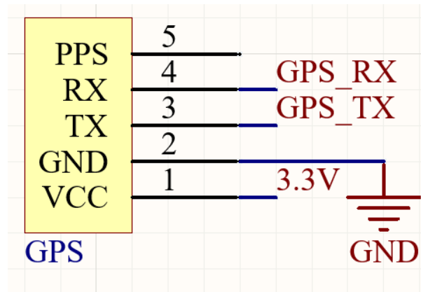
Hình 3.4 Sơ đồ nguyên lý khối định vị GPS ATGM336H
