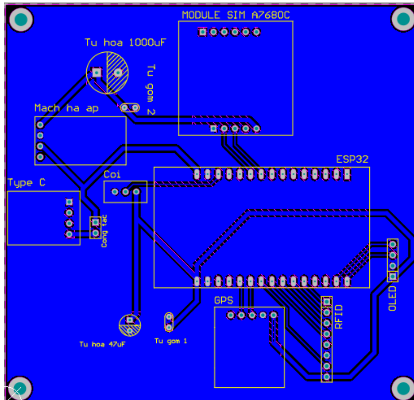
Hình 3.14 Mạch PCB chế độ 2D
