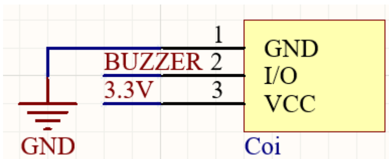
Hình 3.10 Sơ đồ nguyên lý khối thông báo
