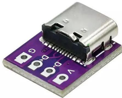
Hình 3.11 Module Type C cái
