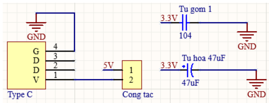
Hình 3.13 Sơ đồ nguyên lý mạch nguồn cấp
