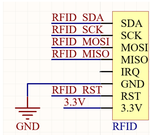
Hình 3.6 Sơ đồ nguyên lý khối RFID RC522
