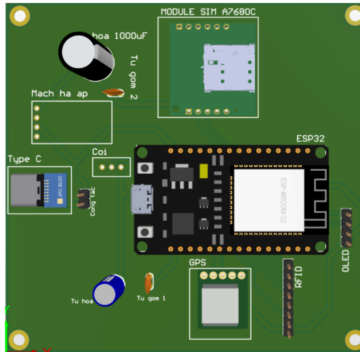
Hình 3.15 Mạch PCB chế độ 3D
