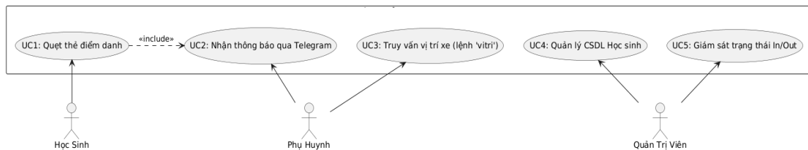
Hình 4.1 Biểu đồ Use Case tổng quát của hệ thống
