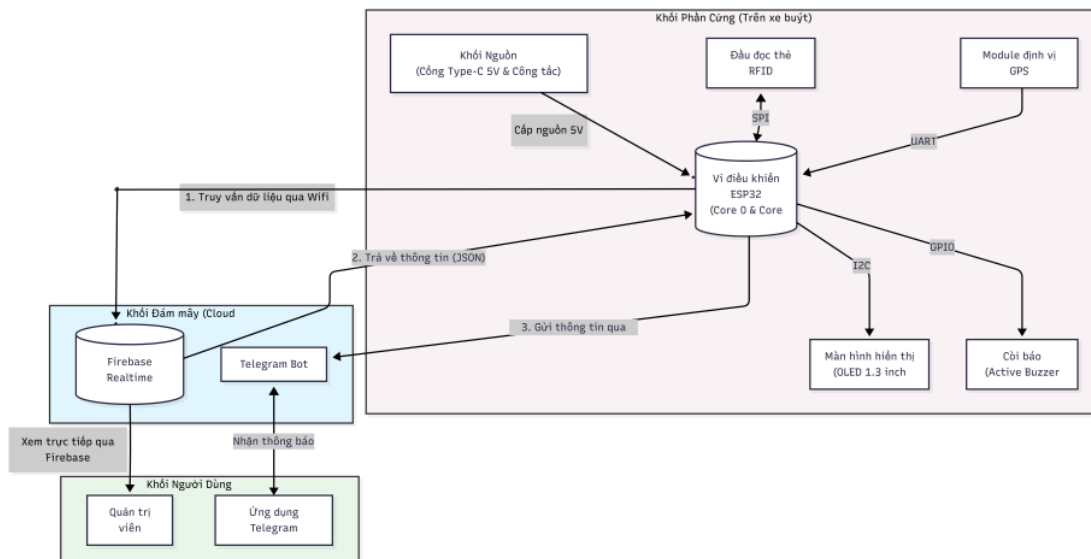
Hình 2.1 Sơ đồ khối kiến trúc hệ thống
