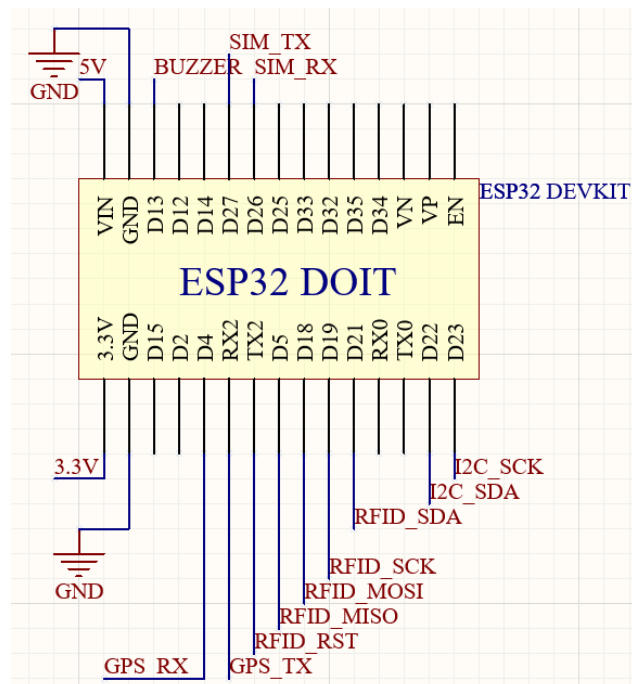
Hình 3.2 Sơ đồ nguyên lý khối vi điều khiển trung tâm ESP32
