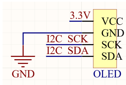
Hình 3.8 Sơ đồ nguyên lý màn hình OLED
