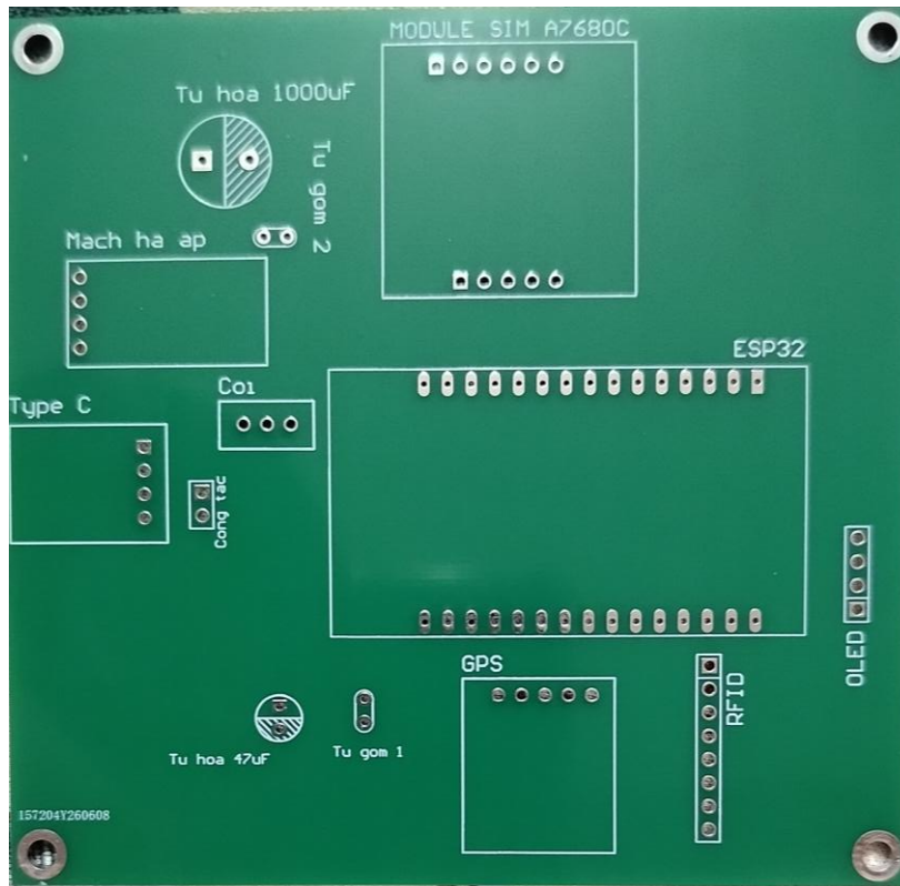
Hình 3.16 Mạch PCB thực tế
