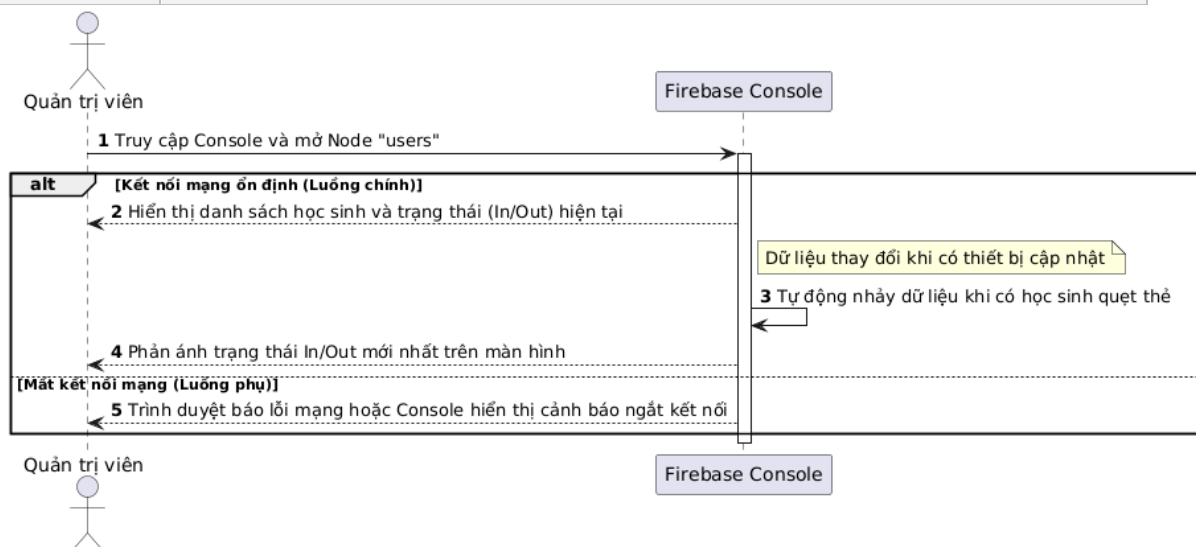
Hình 4.6 Sơ đồ tuần tự của UC5
