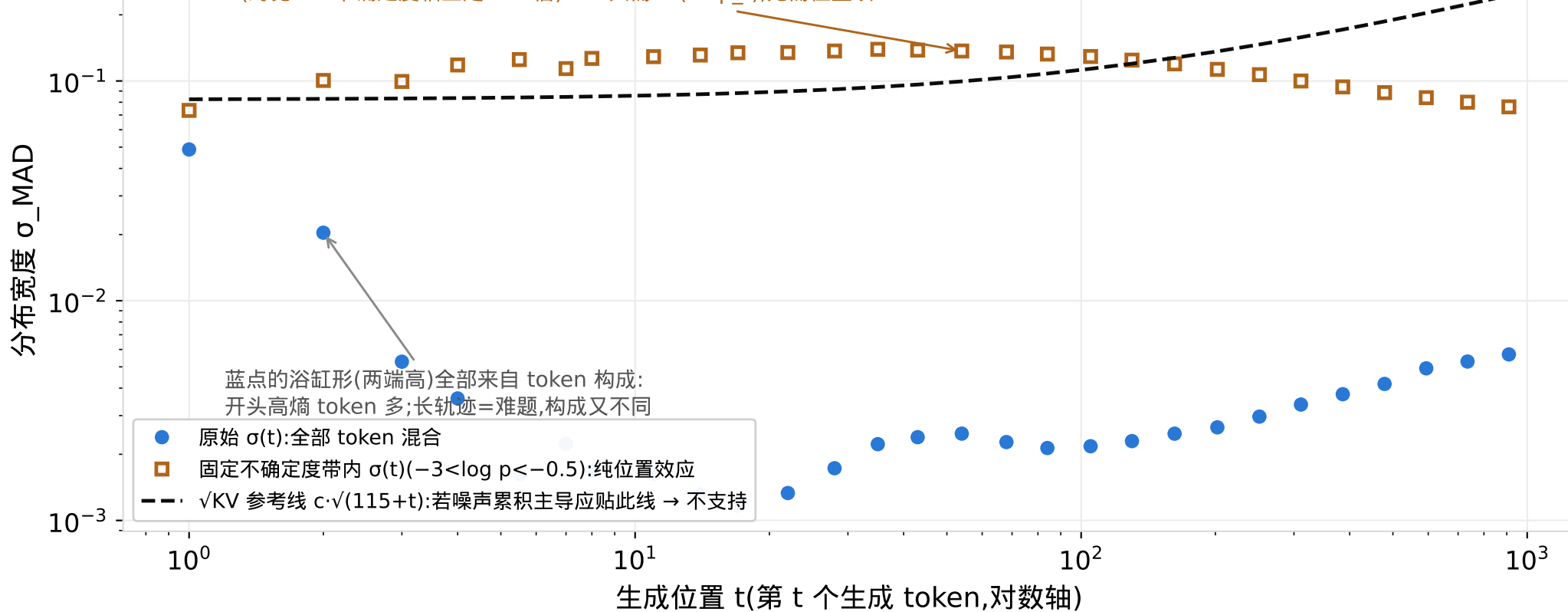
拆解:固定不确定度后 \sigma(t) 近乎平坦 —— 位置不是独立驱动因素
