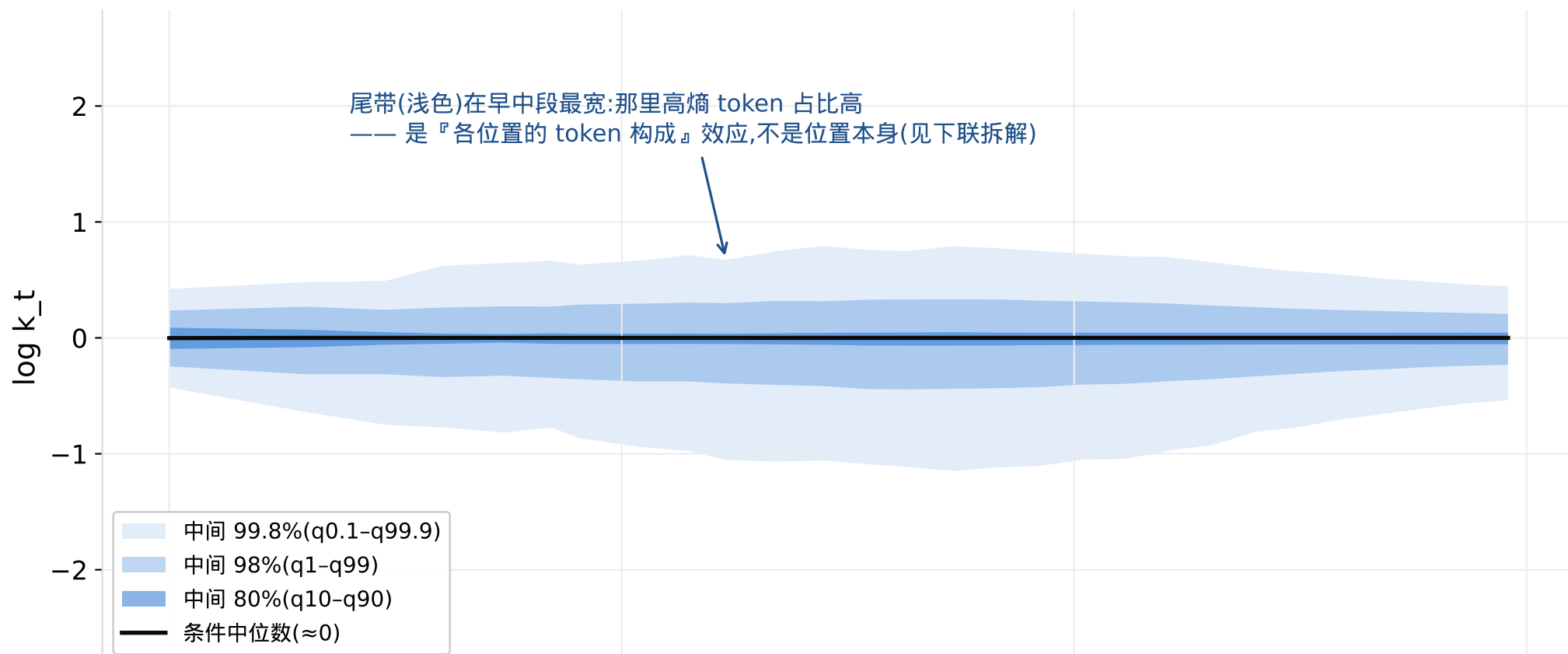
同一生成位置 t 上 \log k_t 的分布(moe, 12,293,115 tokens,2 万条轨迹按 t 汇合)
